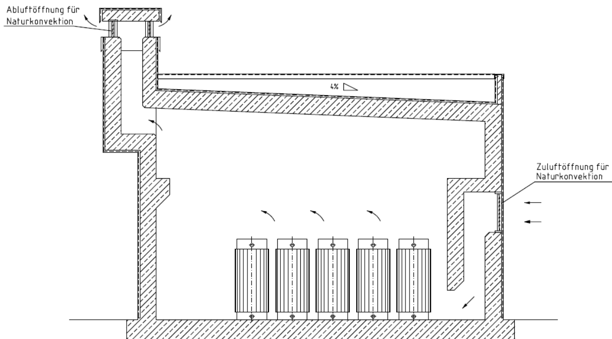
Abb. 14 Wärmeabfuhrprinzip
