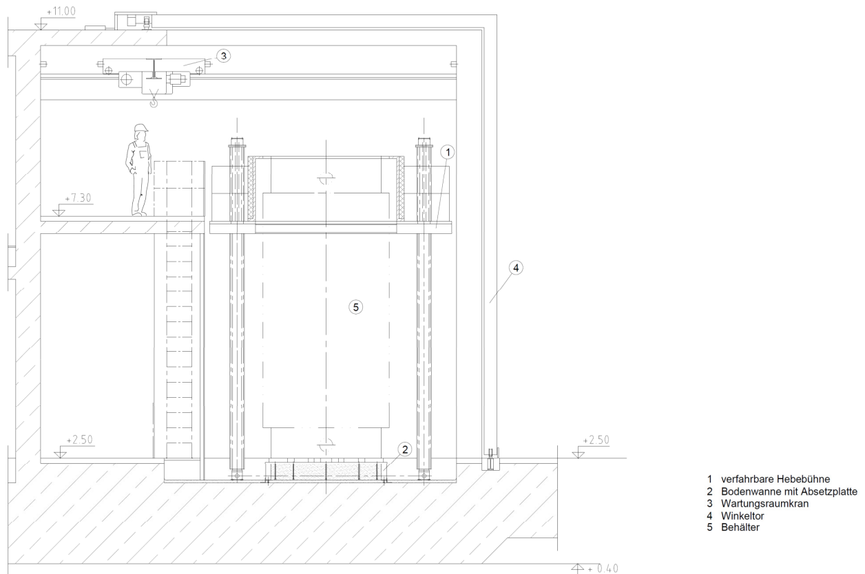
Abb. 13 Übersicht Wartungsraum
