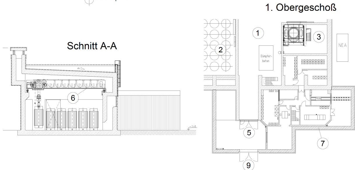
Abb. 12 Übersicht Lager- und Betriebsgebäude
